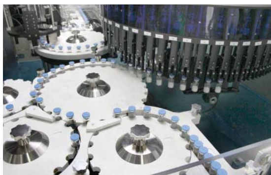
Передача через колеса-звездочки
