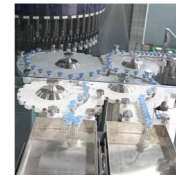
Загрузка флаконов
